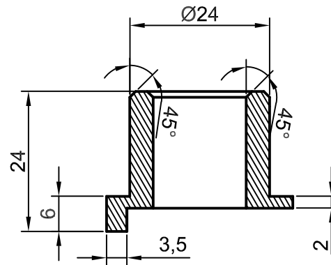
Řez A - A
